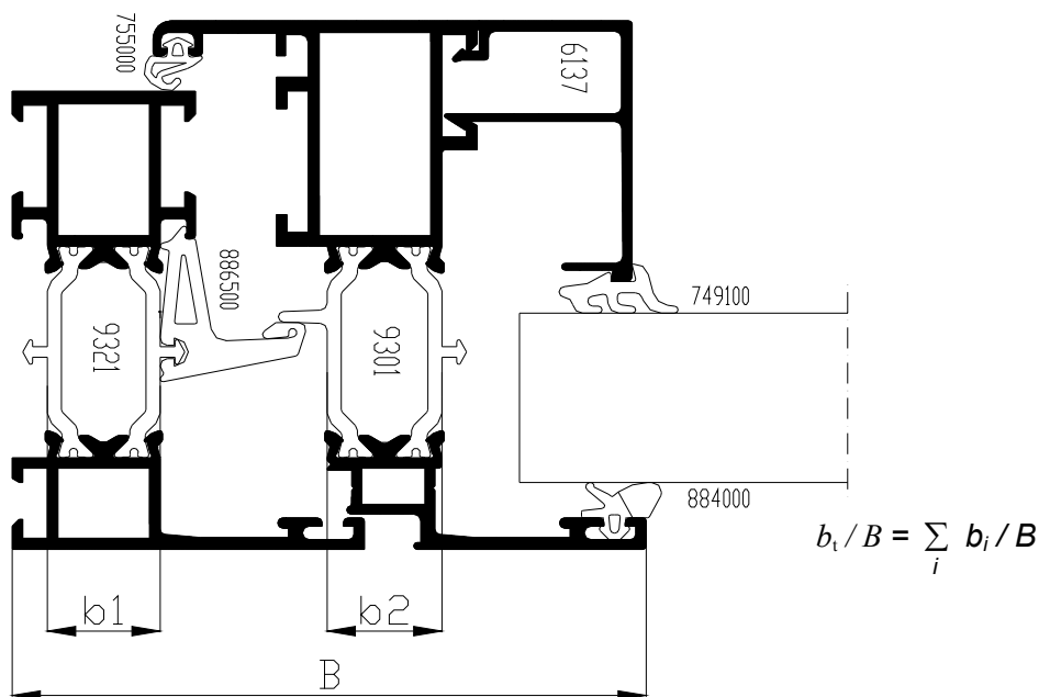
Bild 2 Ermittlung des Verhältnisses b_t / B an den Profilen des Profilsystems 065.
